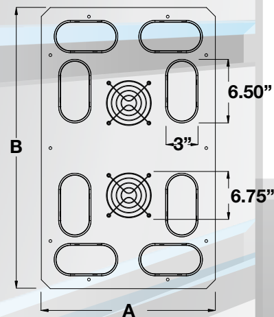
BTA6 Fan
