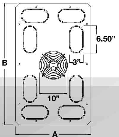
BTA10 Fan
