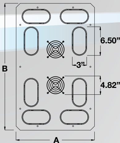
BTA4 Fan
