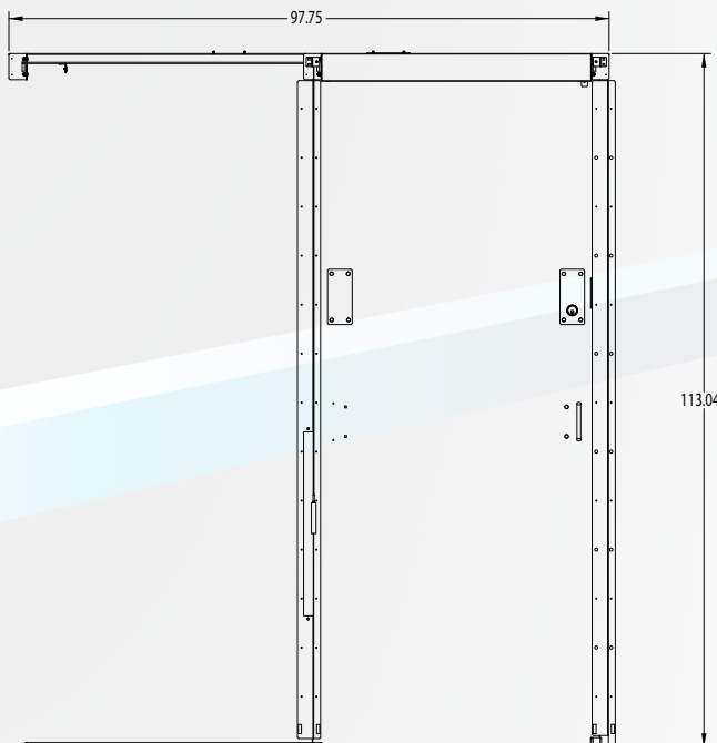
Solid Sliding Door
